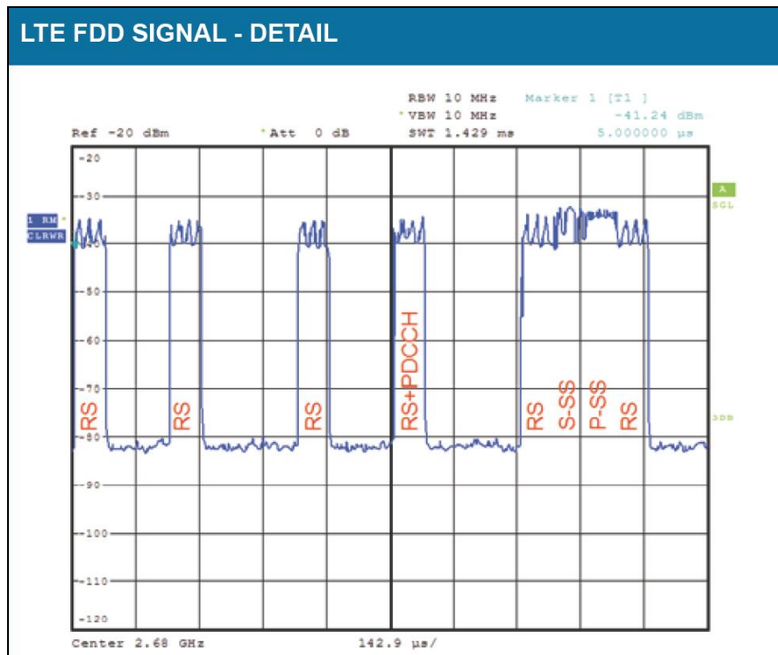
Abb. 6: LTE FDD-Signal im Zeitbereich, ohne Verkehr (Benutzerdaten), Detail aus Abb. 5, auf der horizontalen Zeitachse 142,9 \mu s pro Teilung, Gesamtzeit der Achse 1,429 ms, entsprechend 20 Symbolen (knapp 3 Slots) (Quelle: [5], S. 12)
